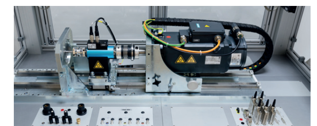
Bsp.-Abb.: Laststrang
