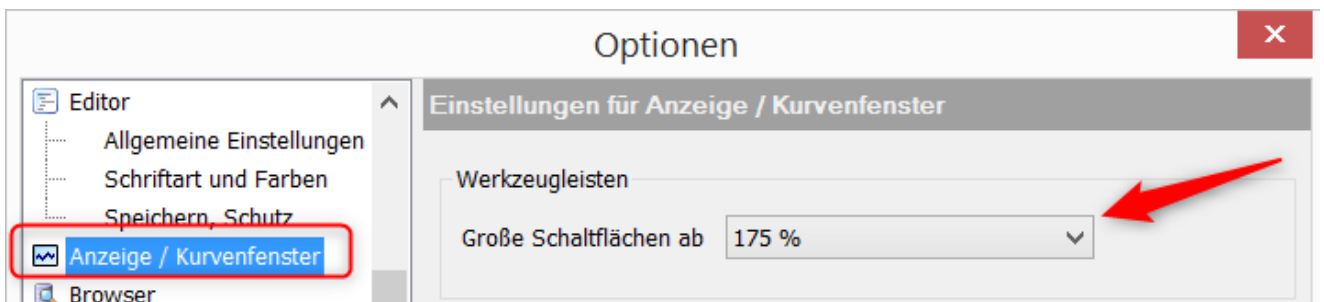
Vergrößerungsfaktor für den Bildschirm, ab dem große Werkzeugleisten verwendet werden.
