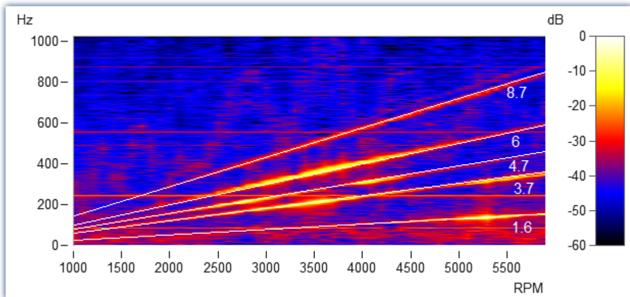
Amplitudenspektrum mit Frequenz über Drehzahl
