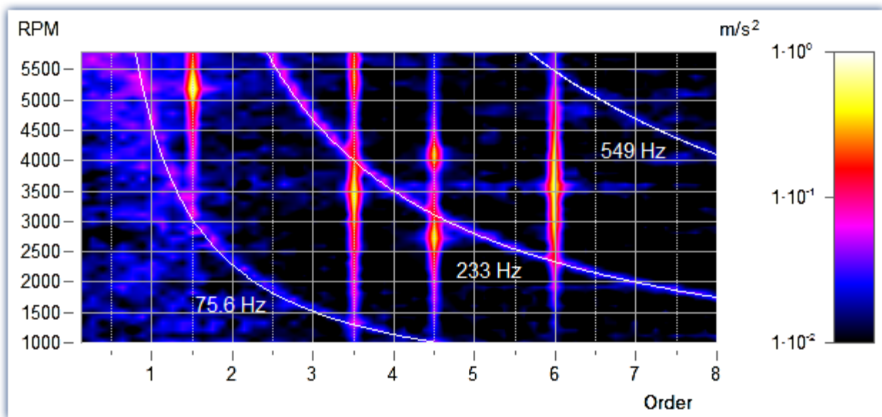
Drehzahl (RPM) und Ordnung
