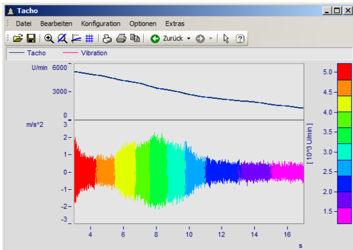
Linienfarbe der Vibration abhängig von der Drehzahl
