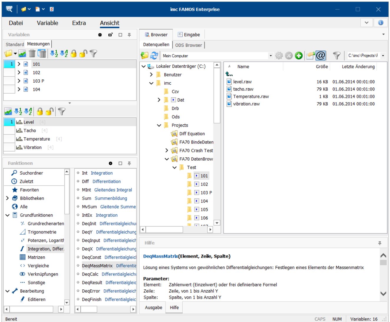
Die Softwareoberfläche präsentiert sich in einem neuen aufgeräumten imc-Look.
